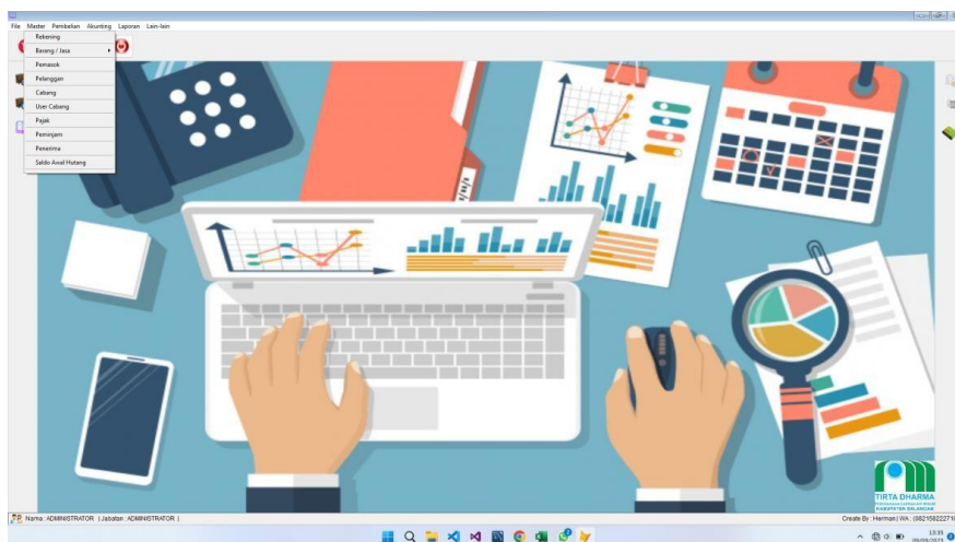
Gambar 1. Menu Utama
